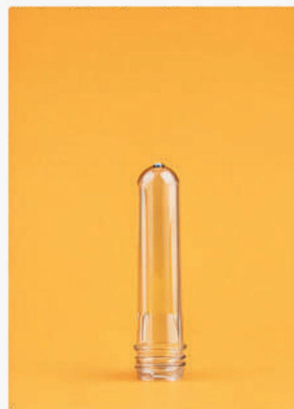
PREFORM D20 Weight | 13 Gram Height | 82 mm
