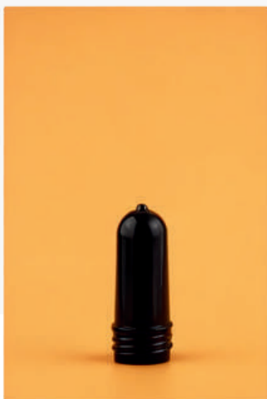
PREFORM D28 Weight | 12 Gram Height | 68.3 mm
