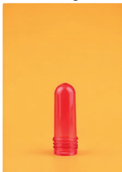
PREFORM D24 Weight | 10 Gram Height | 65.8 mm
